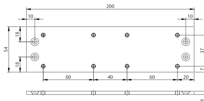
Montážní plech A280
